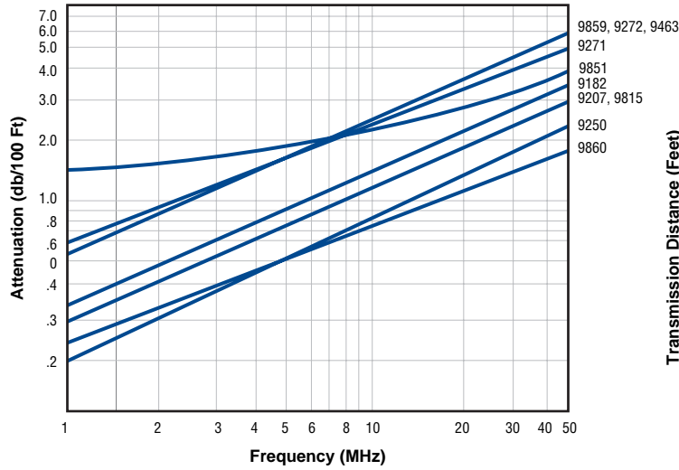
Attenuation
